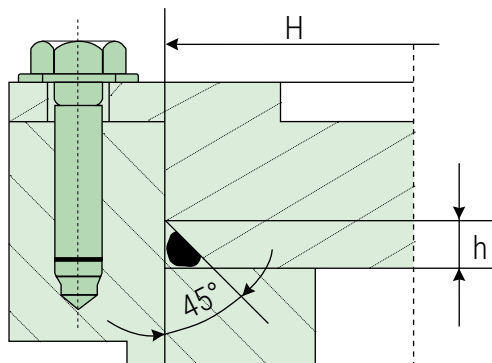
Figura 10: montaggio su coperchio
