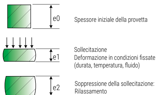
Figura 3: Schema per misurare C.SET
