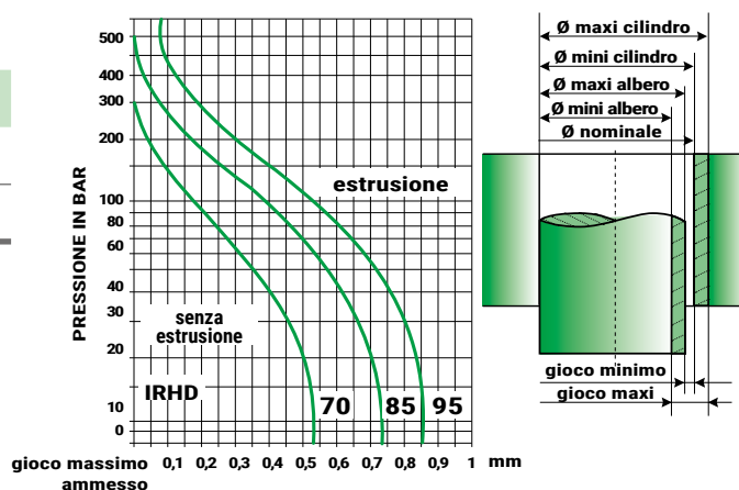
Figura 18: diagramma di estrusione in funzione della pressione, della durezza e del gioco meccanico:
