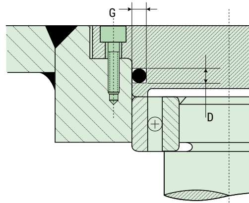
Figura 12: sede aperta all'esterno
