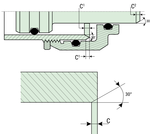
Figura 9 : smussi di invito
