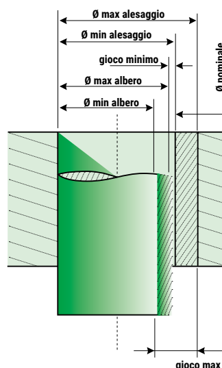
Figura 15: tolleranze e accoppiamenti
