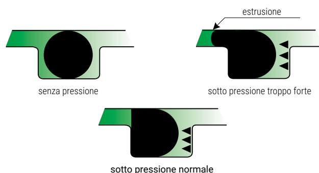
Figura 17: estrusione di una guarnizione
