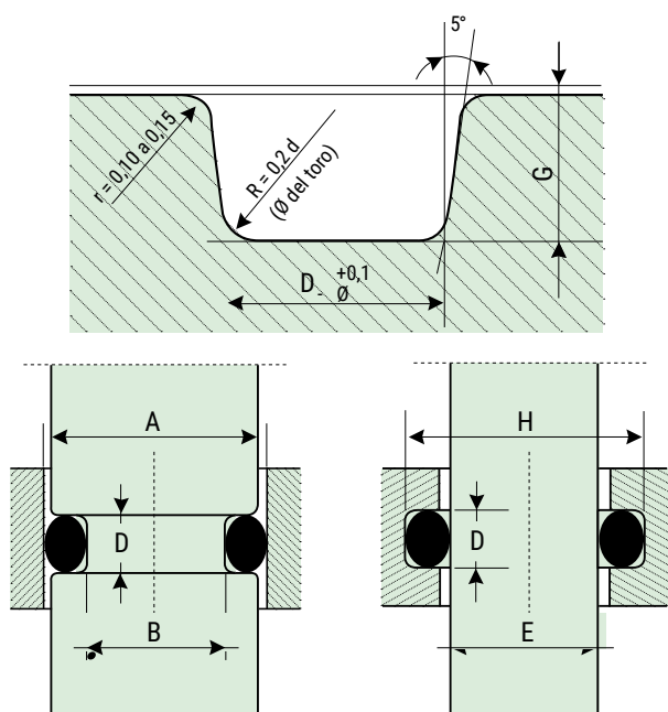
Figura 14: descrizione sedi per applicazioni in movimenti alternativi
