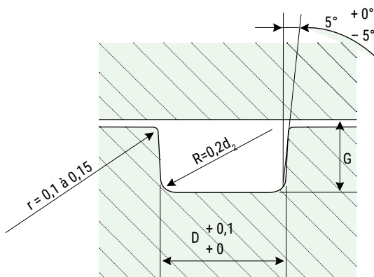
Figura 5: descrizione di una sede rettangolare
