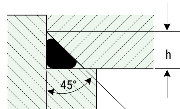
Figura 6: descrizione di una sede triangolare
