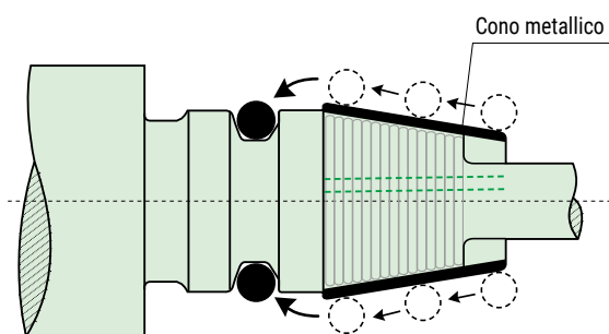
caso 1: protezione contro filettatura interna
