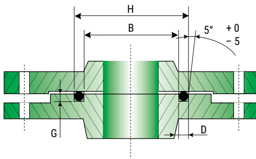
Figura 11: montaggio su flange
