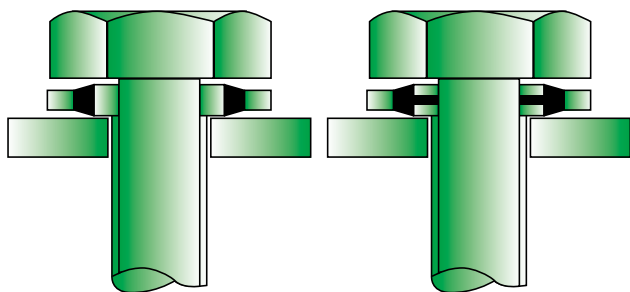
BS standard e versione autocentrante
