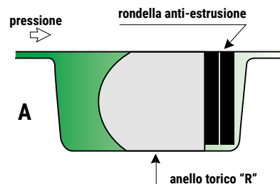
Figura 20: esempi di montaggio di anelli torici con rondelle antiestrusione
