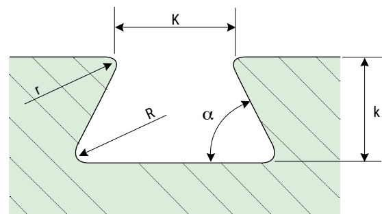
Figura 7: descrizione di una sede trapezoidale
