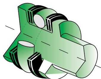
esempio di montaggio di anello torico "R" con due rondelle anti-estrusione, secondo standard MS - 28.782
