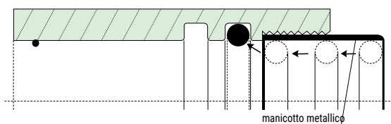
caso 2: protezione contro filettatura interna
