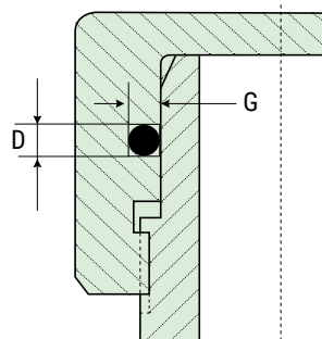
Figura 13: sede aperta all'interno
