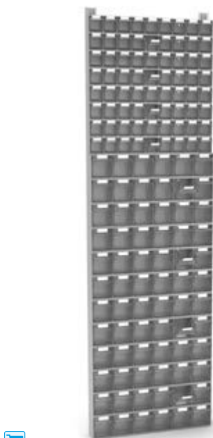
SCAFFALE CON 144 CASSETTI VISUAL BOX DIM. (mm): L=602 P=114 H=2000
